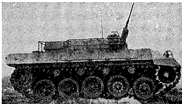
עיקר השוני שב-M-39 (ארה"ב — נהוג בצבא מערב-גרמניה עכשיו) לעומת זחלמי מלחמה 2 הוא בהיותו זחליל-שלם — אך עודו פתוח.
