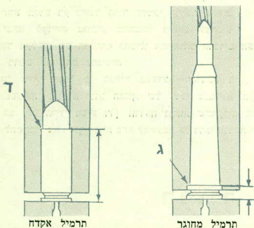
מידות הרחק ראש-תחמיש
