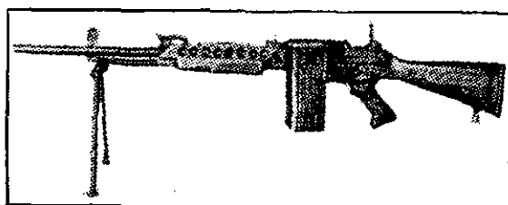
מקלע קל - מוזן-סרט
