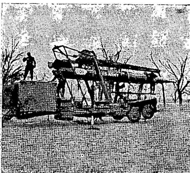
11. ארבעה ברגי חיבור מהיר מצמידים את ראש הנפץ אל מערכת ההנחיה; בו"בזמן מור" כבות מערכות משטח ההיגוי אל המנוע.
