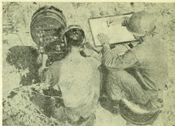
"הזקיף האילם", מכשיר המאפשר לרגלי תצפית אף במזג אוויר גרוע או בחשיכה — מוצב כאן בעמדה פתוחה. "מספר שנים" נראה מסמן בלוח את מהלך התצפית.
