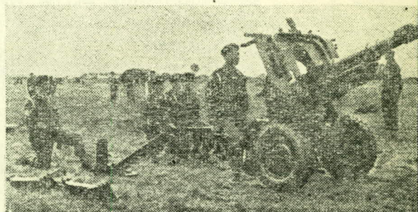
הוביצר-המעמס הבריטי החדש, ב-105 המ"מ, מוצב לירי ככלי-ארטילרית-שדה
