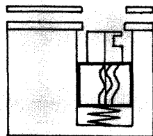
כ. טובלן התאוצה ברחיצה לאחור, במצב ירי רגיל
