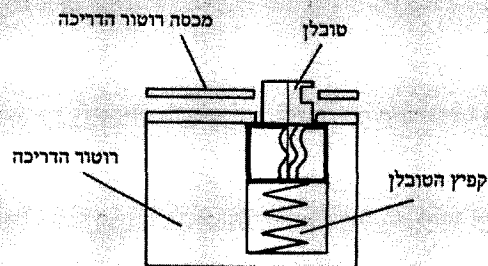
א. מערכת דריכה במצב נצור
