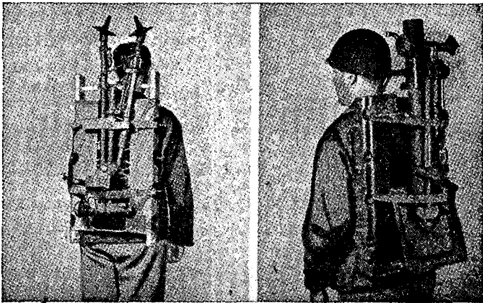
לוח-המשא נוסח יוקון עשוי עץ ואליו מחובר דורגל למרגמת 81 מ"מ.
