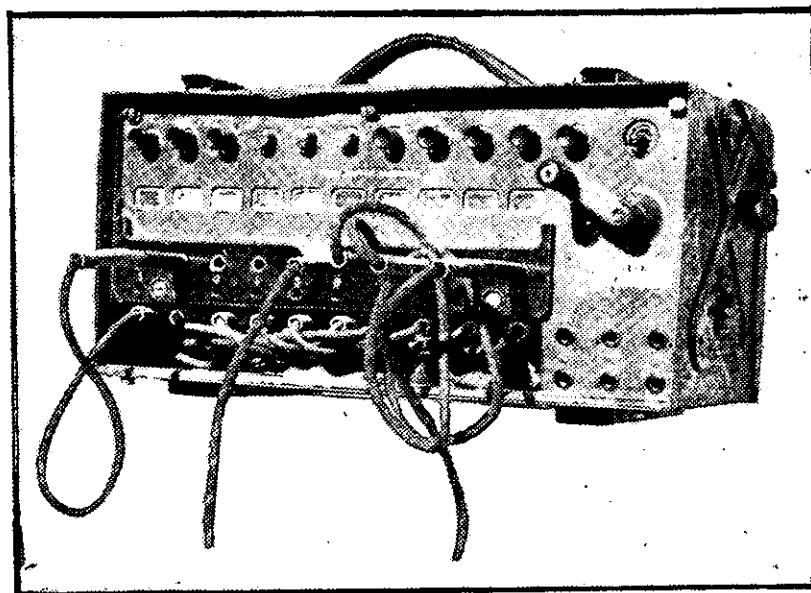
מרכזית שדה צ'כית TU-11
