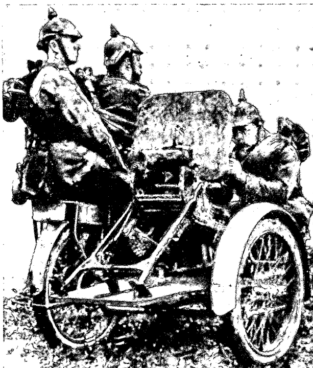
אופנוע עם סירת צד ומקלע בינוני מתוצרת נס.א. (1915)
