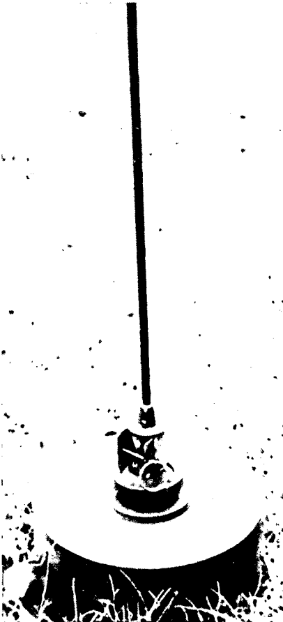
מוקש ג"ט כבד מסוג M-21 פועל כמוקש-לחץ או כאשר מוט האנטנה מתכופף בשיעור של 20 מעלות.
