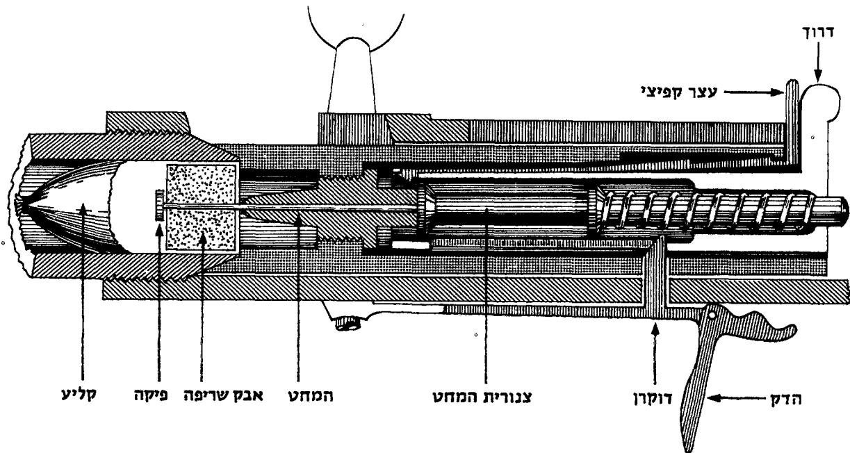
רובה המחט הפרוסי „דרייזר“ — חתך
