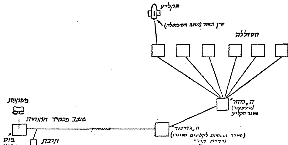
תרשים טכני של מערך סוללת קליעי .ס.ט. 10" ואורח הפעולה
