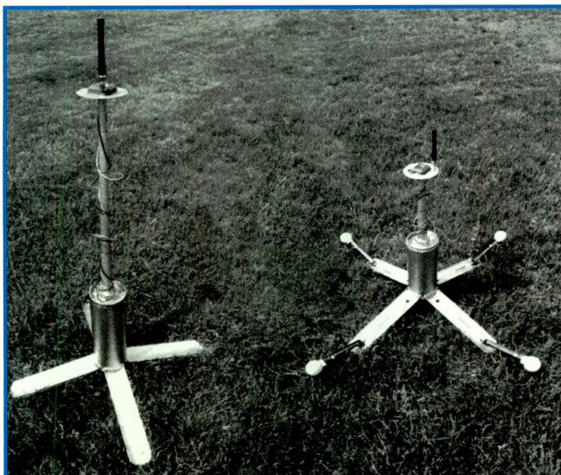
חישנים אקוסטיים-סייסמיים עם "גיי-פי-אס". החישן השמאלי משמש כ"צומת" תקשורת: הוא אוסף מידע מחישנים סמוכים ומעביר אותו אחורנית למפקדה
