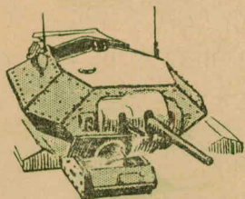
"צריח היהלום" האפייני של טנקי-סיוור בריטיים ("קרוסיידר", מהטיפוס) הישן יותר, בעל תותח בן 2 ליטראות. התר- ניט — על הצריח ועל תאן האחורי.
