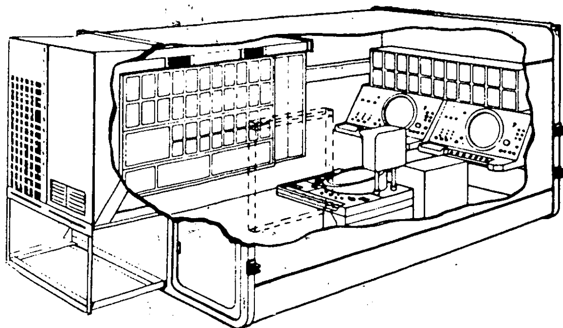
מִרְכֵּז־הַבִּקְרָה הַסּוּלָלִית. הוֹדוֹת לִקְלוֹת מְבִנְהוּ, אִפְשָׁר לְהַעֲבִירוֹ בַּמִּשְׁאִית אוֹ בַּהֲלִיקוֹפְטֵר. כָּל הַצִּיּוֹד הָאֶלֶקְטְרוֹנִי הַדּוּוֹשׁ כָּלוֹל בְּתוֹכּוֹ.
