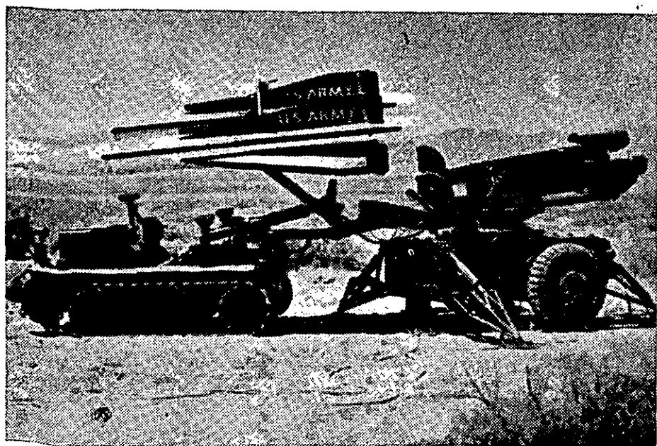
רִכְב־הַטְּעֵנָה זַחְלִי הַמְּסוּגֵל לְהַטְעִין אֶת כֹּן־הַשִּׁיגוֹר תוֹךְ שְׁנֵי מִסְפָּר. לֵאחֲרַי הַטְּעֵנָתוֹ מְשׁוּעֵבֵד הַכֹּן לַמִּכָּ"מ־הַמַּאֲיִר וְזוּיּוֹת הַכִּיּוּן נִקְבְּעוֹת בּוֹ לִפְנֵי שִׁיגוֹר הַסִּיל.
