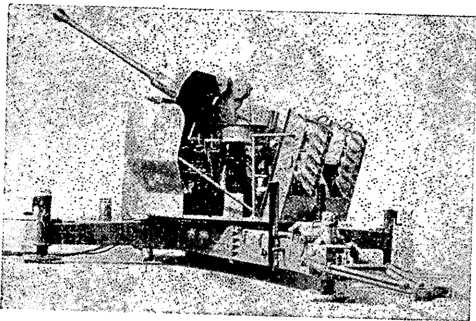
תותח נ"מ בינוני "Bofors" בן 40 מ"מ
