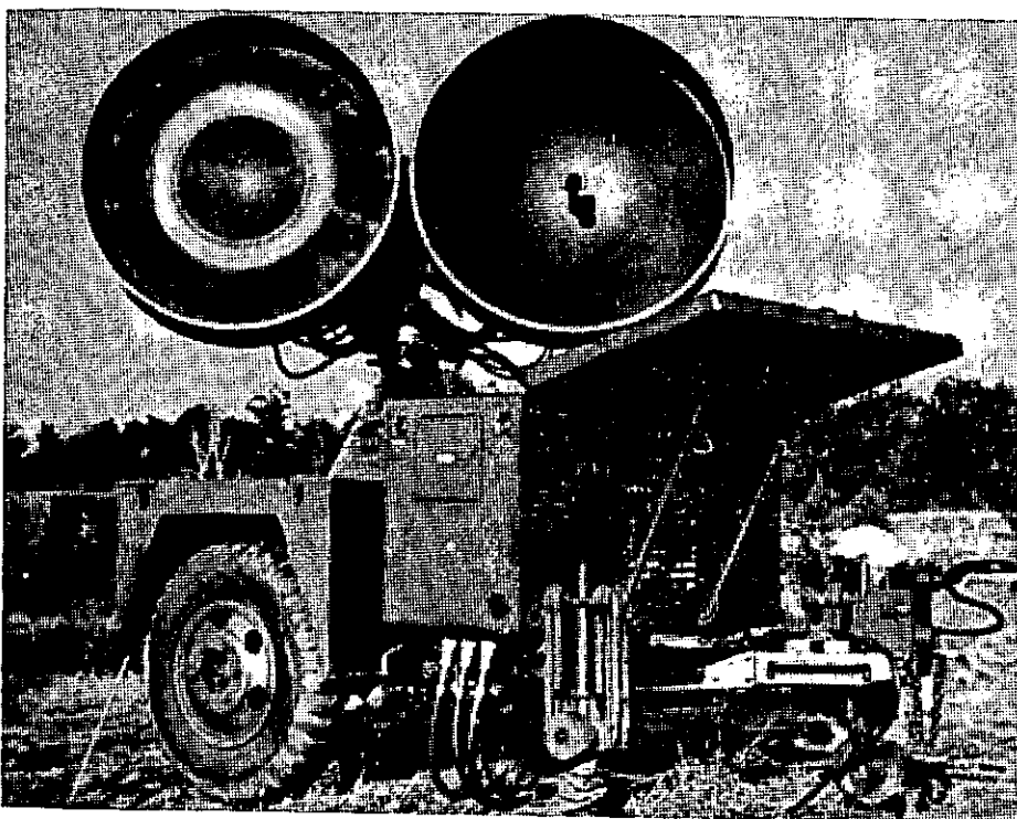
כְּמוֹ יַחֲדוֹת הַמִּכָּ"מ הָאֲחֵרוֹת מוֹרְכָבִים שְׁנֵי הַמַּאֲיִרִים עַל גִּרְוֵרִים דְּרִאוֹפְנִיִּים. בַּתְּמוּנָה נִרְאֶה מִכָּ"מ־מַאֲיִר בַּעַל עֲצֻמָּה נִמּוּכָה.
